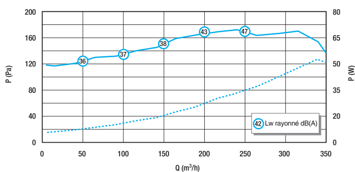
Courbe aérodynamique et acoustique EasyHOME Hygro Compact Premium HP+
