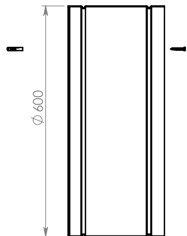
SECTION D-D SCALE 1 : 10
