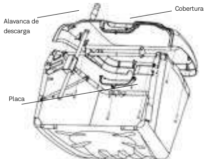
Cobertura
