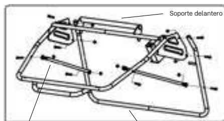
Soporte lateral
