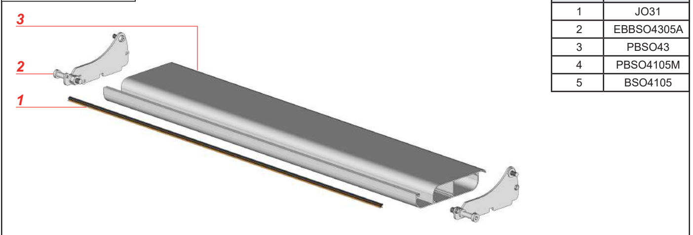
Lame orientable.
