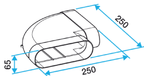
Coude horizontal 90°
