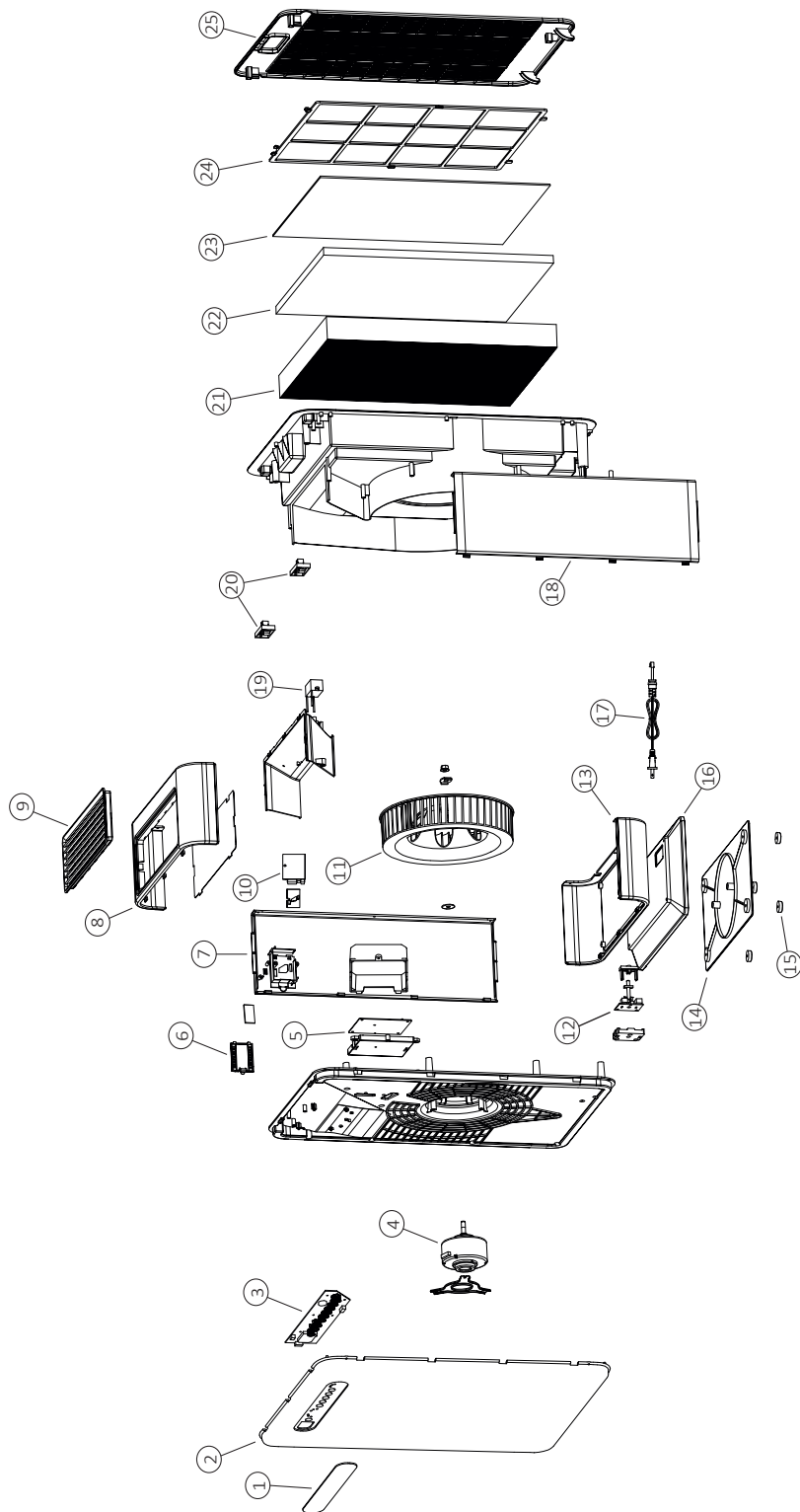
Fig. 18: Vue éclatée LRM 350, LRM 500
