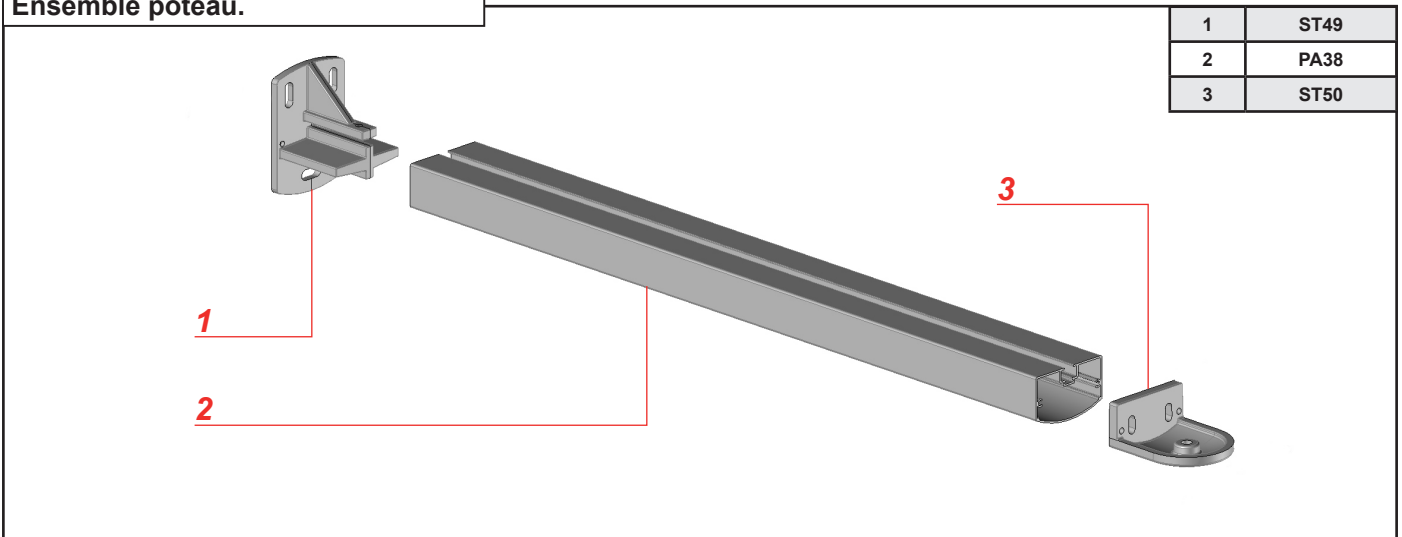
Ensemble poteau.
