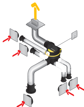
Installation kit ColorLINE avec conduits souples Algaire
