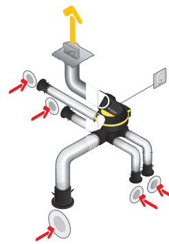
Installation kit BIP avec conduits souples Algaire
