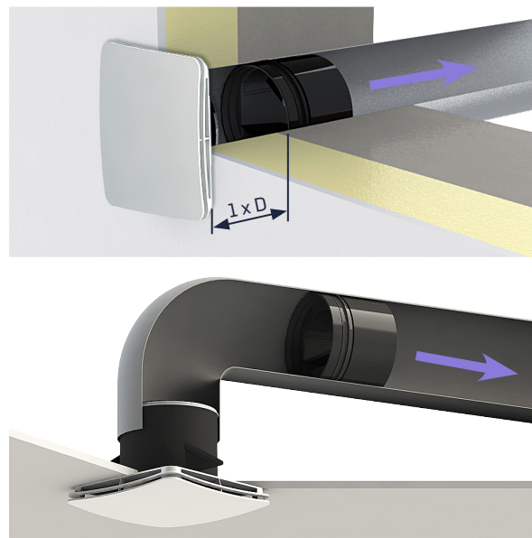
AURÉA avec régulateur de débit RDR en extraction
