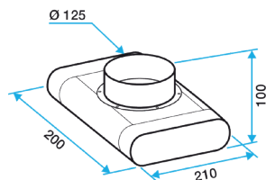
Té 90° vertical pour bouche
