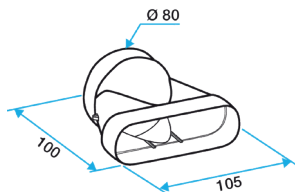
Raccord mixte pour conduit Ø80 mm
