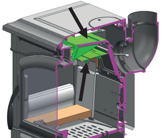
2 - DÉFLECTEUR DE FUMÉE
