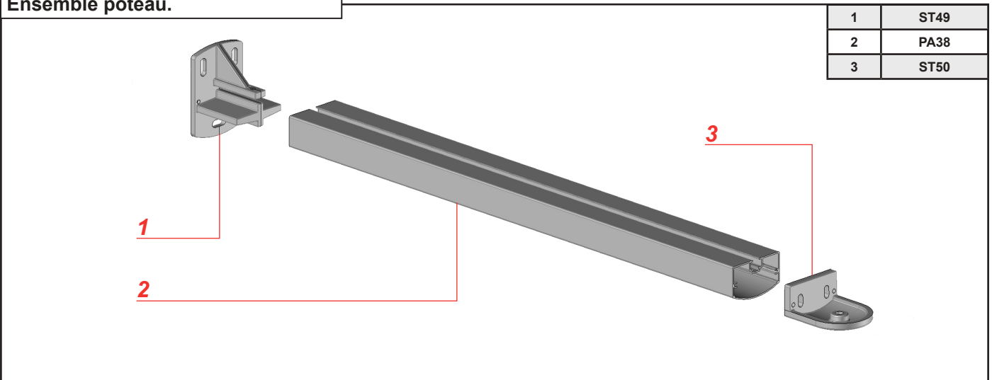
Ensemble poteau.
