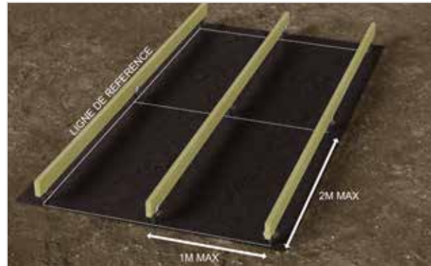
Exemple pour structure croisée en bois avec solives 45 x 145 mm et lambourdes 45 x 70 mm
