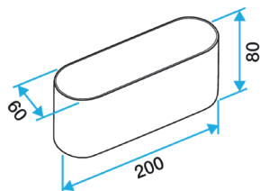
Raccord mâle 60x200 mm
