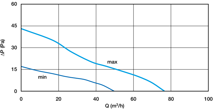
Courbes aérodynamiques INEA 100
