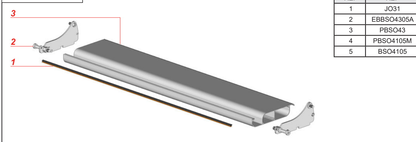
Lame orientable.
