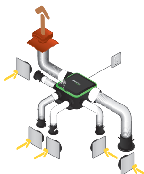
Installation avec conduits souples Algaie
