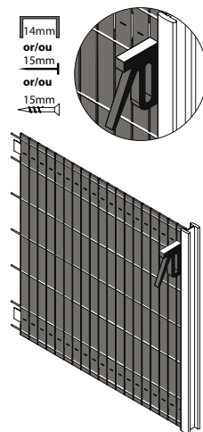
3 - Glissez ensuite toutes vos lames dans les mailles jusqu'au remplissage du panneau en évitant de les faire toucher le sol.
