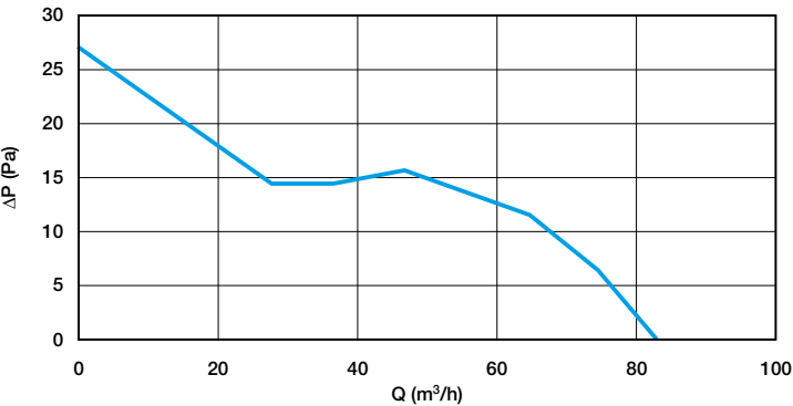
Courbe aéraulique GRAPHIC 100
