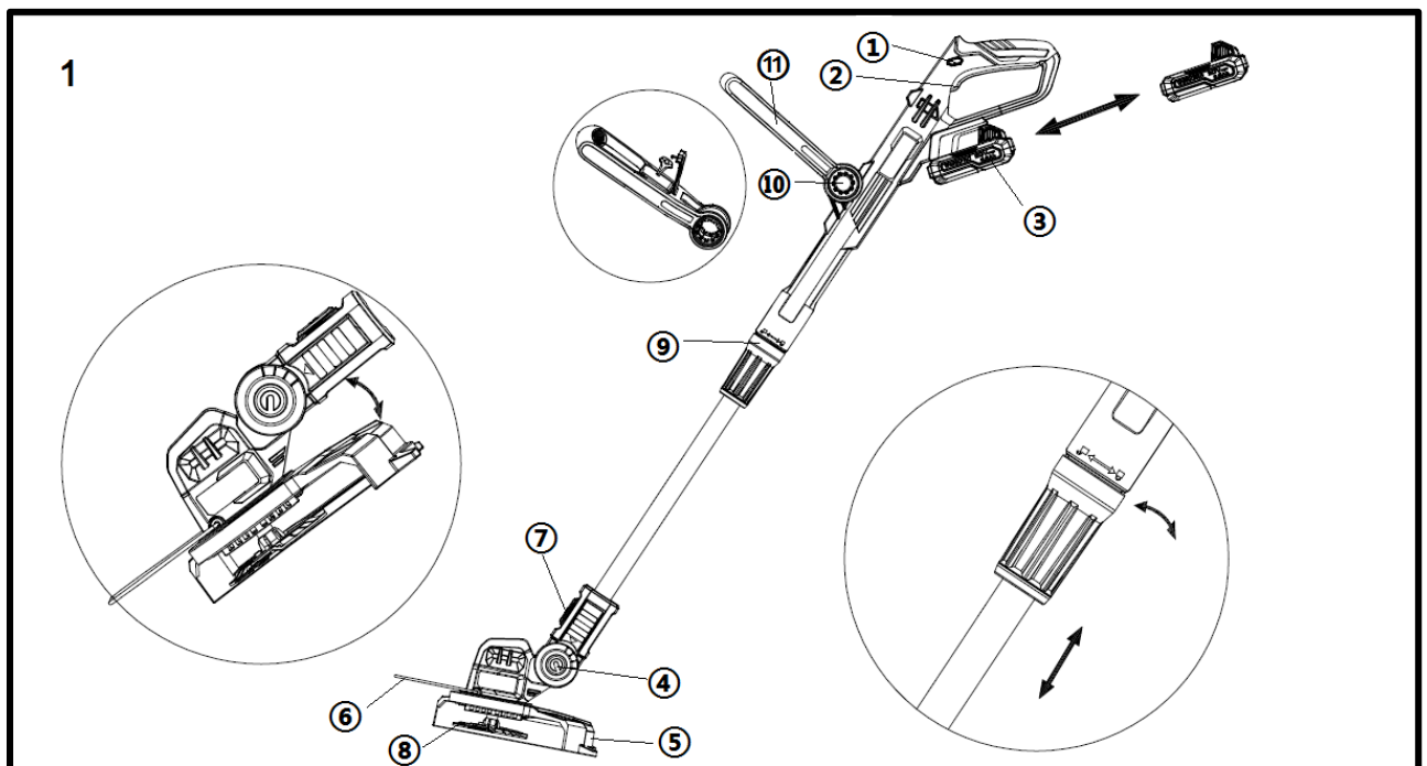
Bild 1: Grästrimmer
