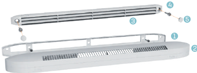
Montage sur entaille 250 x 15 ou 250 x 12 mm
