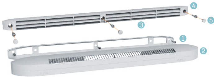
Montage sur entaille 354 x 12 mm
