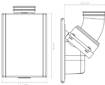
Encombrement prise pour flexible rétractable
