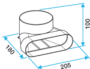
Coude 90° vertical pour bouche
