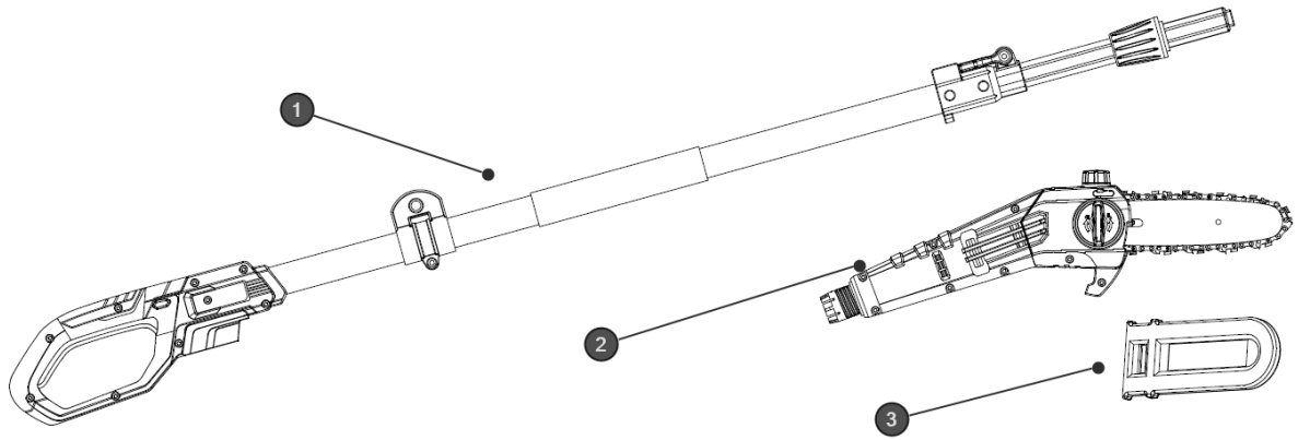
Figura 1: Podadora de pértiga
