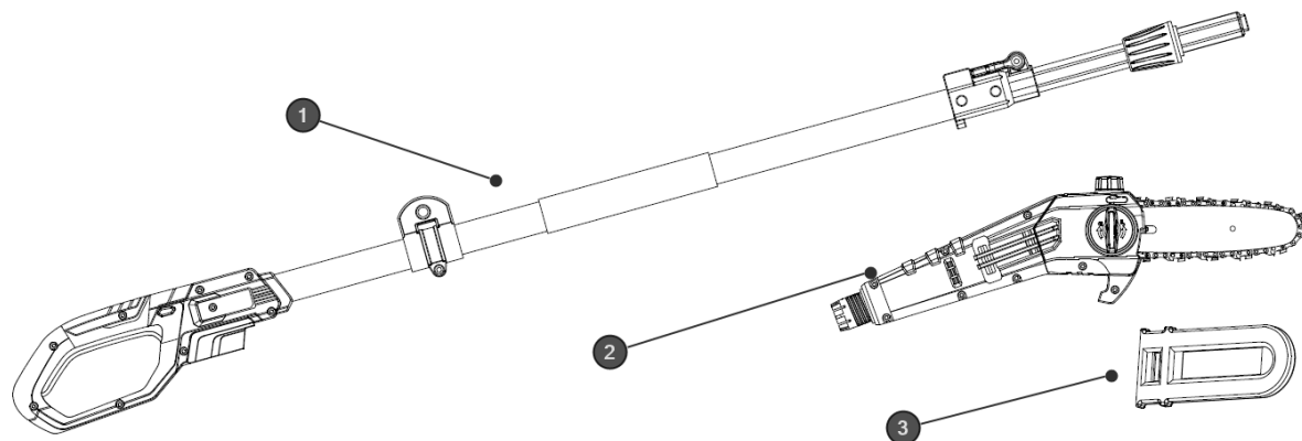
Figura 1: Potatore ad asta
