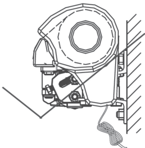
INSTALACJA PRAWIDŁOWA
