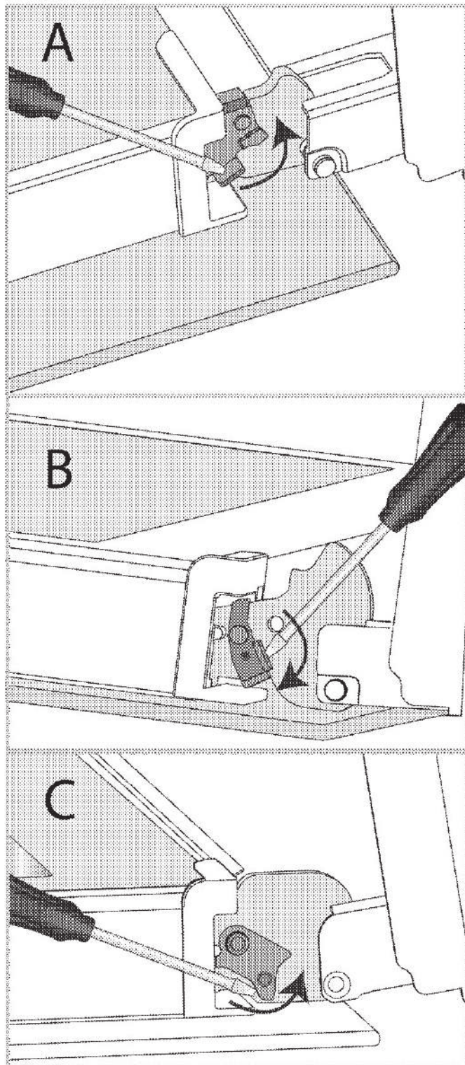
Verrouillage de charnière - position fermée
